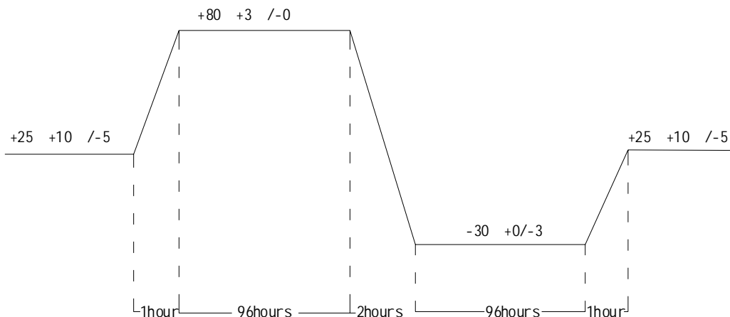
FIG1 TEMP. TEST
